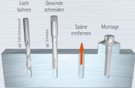
Prozesskette bei Einsatz einer metrischen Schraube.
